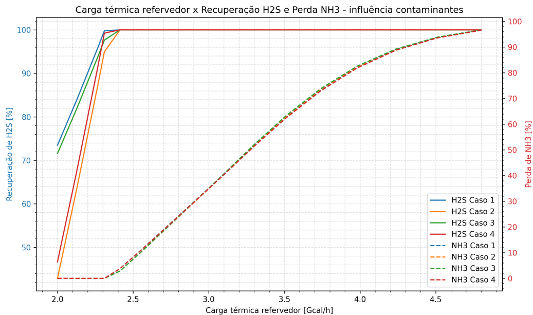
Figura 3: Carga térmica x recuperação de \text{H}_2\text{S} e perda de \text{NH}_3
