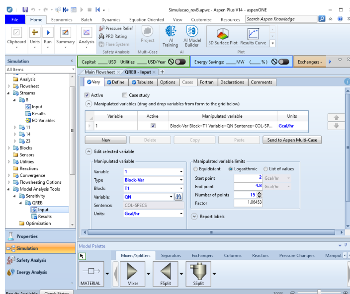
Figura 2: Ferramenta da análise de sensibilidade do Aspen Plus
